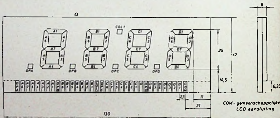
Fig. 4c. IEE - LCD, type 1504 - 03 (T) of type 1604 - 03 (R).
