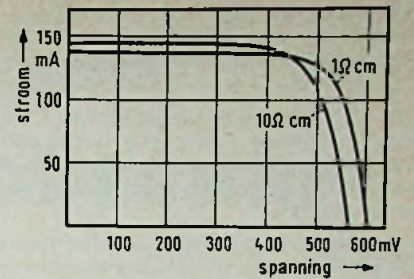
Fig. 7 Stroom/spannings-karakteristiek voor 1 en voor 10 Ω cm cellen.
