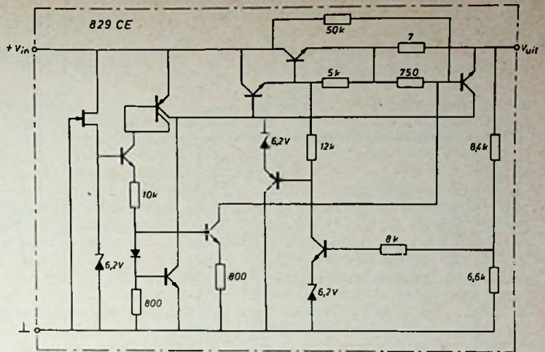
Fig. 6a. Principe van de Teledyne 12 V spanningregelaar.
