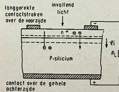
Fig. 2 Doorsnede van een zonnecel.
