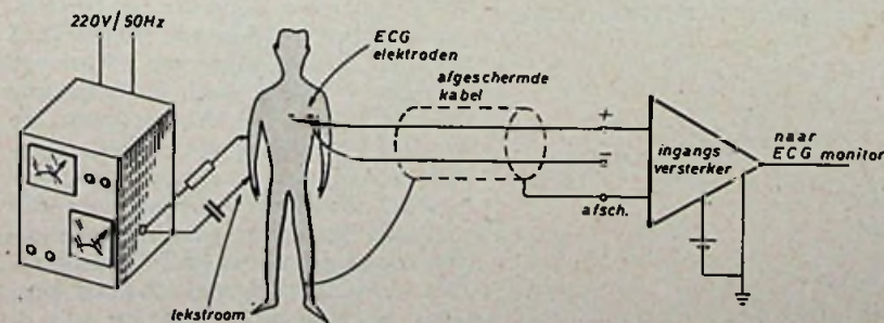
Fig. 6 In medische toepassingen, waar patienten in contact kunnen komen met slecht geaarde apparatuur, worden lekwegen effectief verbroken door gebruik te maken van isolatieversterkers, waardoor elektrocutie van de patient wordt voorkomen. In vele gevallen hoeft de fatale stroom maar enkele \mu A groot te zijn om de patient te kunnen doden.
