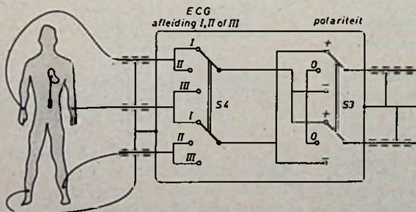
Fig. 4 Instelling van de verschillende afleidingen.
