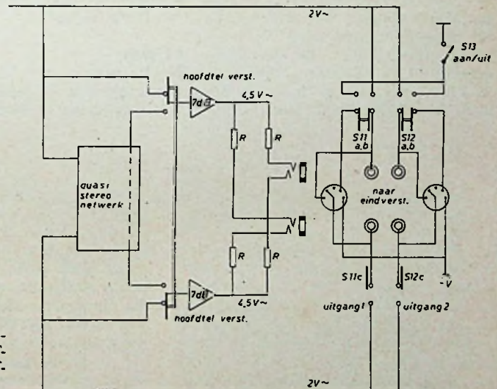
Fig. 11. Blokschema van het LF-deel van de afstemmer.
