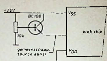
Fig. 3. Helderheidsregeling.
