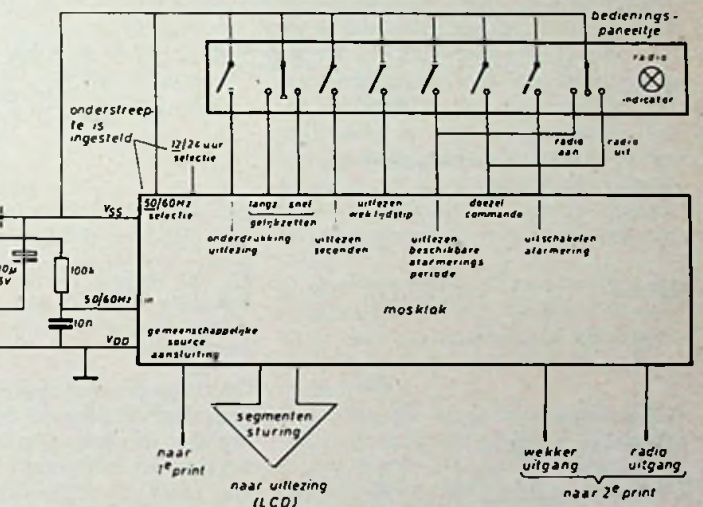
Fig. 7. Aansluitgegevens van de MOS klokchip.
