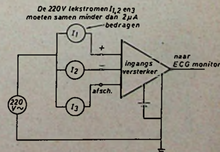
Fig. 6 In medische toepassingen, waar patienten in contact kunnen komen met slecht geaarde apparatuur, worden lekwegen effectief verbroken door gebruik te maken van isolatieversterkers, waardoor elektrocutie van de patient wordt voorkomen. In vele gevallen hoeft de fatale stroom maar enkele \mu A groot te zijn om de patient te kunnen doden.
