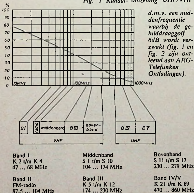
Fig. 1 Kanaal-omzetting UHF/VHF
