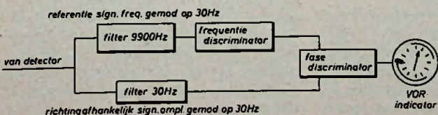
Fig. 20 VOR-deel in de navigatie ontvanger.
