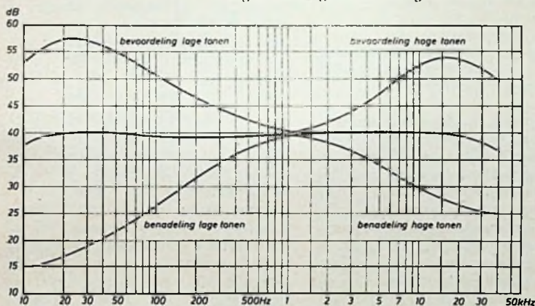
Fig. 5 Frequentiearakteristiek als functie van de klankregeling.
