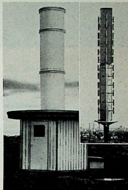
Afb. 21 Een compleet VOR solide state bakken (ITT) met in de inzet afb. 22, een DME antenne.
