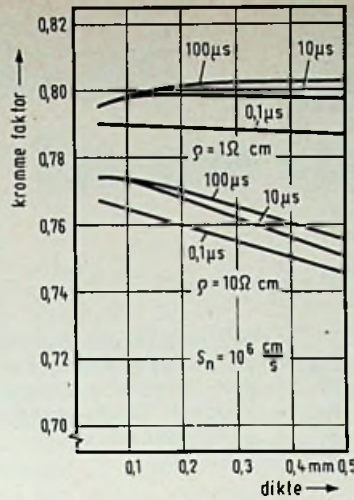
Fig. 9 Kromme-factor als functie van de dikte van 1 en van 10 \Omega \cdot \text{cm} cellen.
