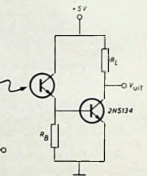
Fig. 1. Optische koppeling met impulsversterker, algemeen schema voor de MCT9.
