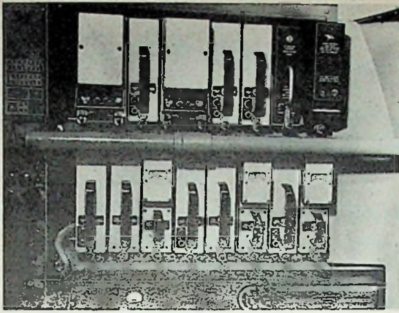
Afb. 23 Het radio rek uit de Trident met op het bovenste rek, twee VHF zenders, drie VHF ontvangers, intercom versterker en cabine omroep-versterker, daaronder weer drie VHF ontvangers met bijbehorende navigatie units en twee glide-slope ontvangers. Deze serie behoorde tot de eerste bijna geheel getransistoriseerde apparatuur die o.a. voor de eerste CAT III landingen werd toegepast. (Marconi Ltd).
