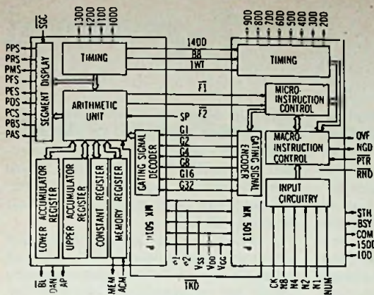
Blokschema en aansluitgegevens der beide circuits.
