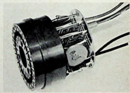
Foto vermenigvuldiger met 1% weerstanden in epoxy omhulling.
