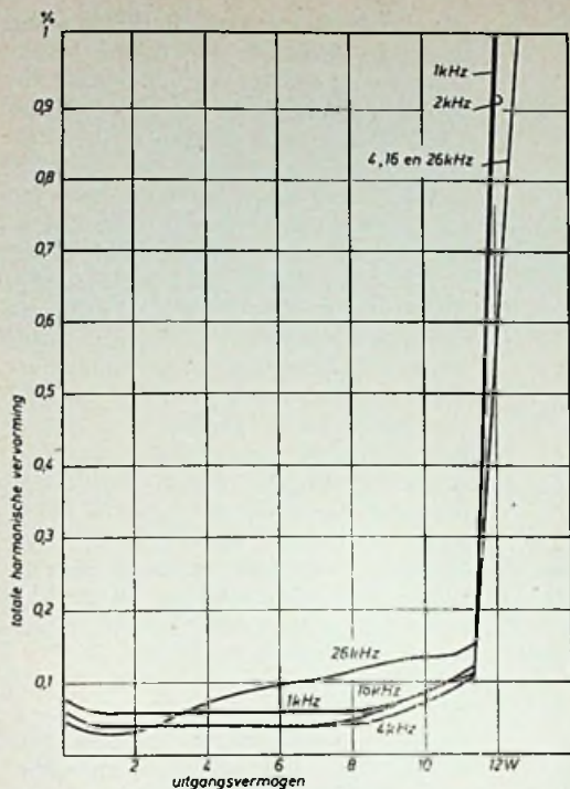
Fig. 6 Harmonische vervorming van de versterker bij gebruik van een niet-gestabiliseerde voeding.
