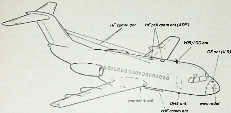
Fig. 28 Eén van de vele mogelijkheden van antenneplaatsing.
