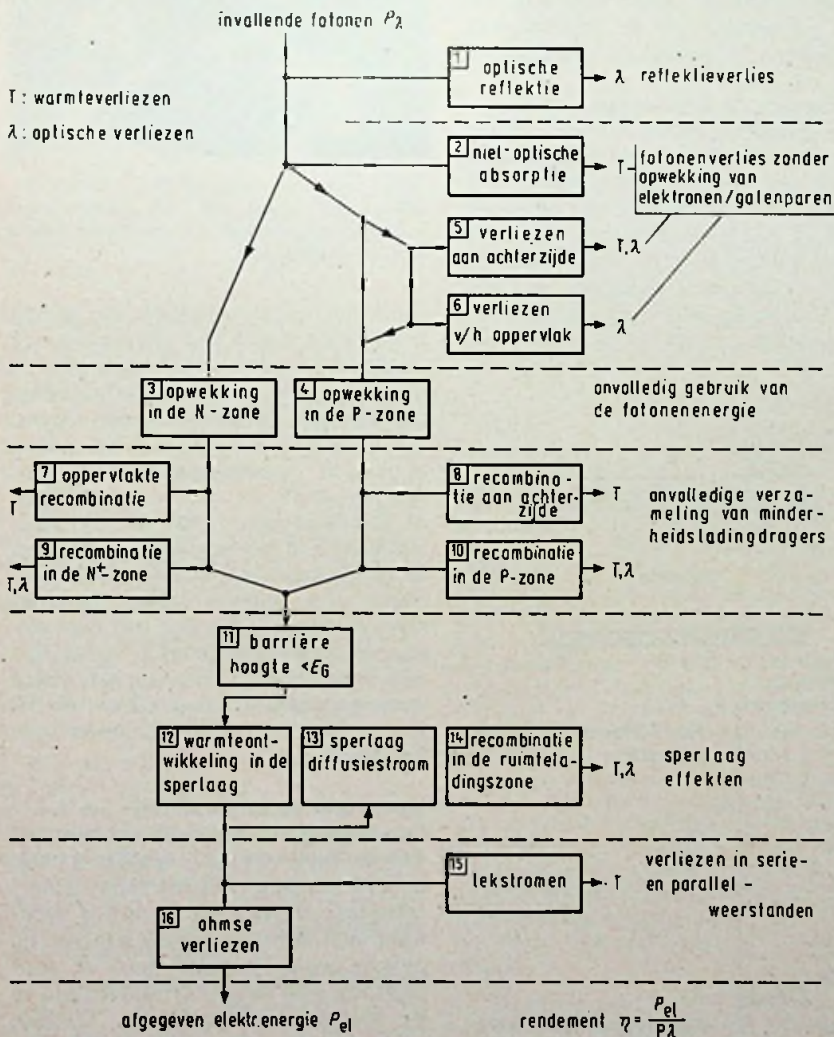
Fig. 5 Verliezen bij licht-elektrische energieomzetting.
