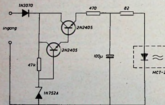
Fig. 6. Verbeterde schakeling van het ingangscircuit van fig. 5.
