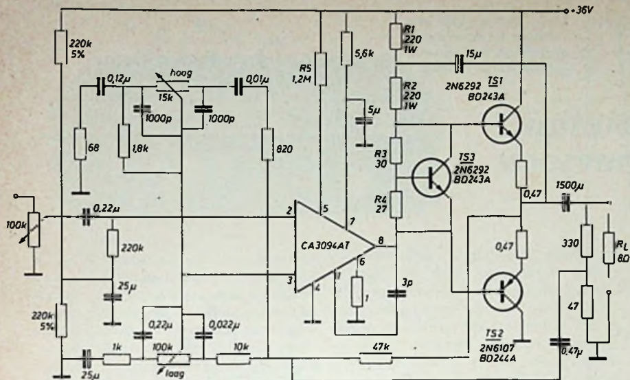
Fig. 4 Vermogenversterker, gevoed uit één voedingsbron.
