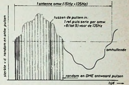
Fig. 25 Antenne patroon van het TACAN bakken.
