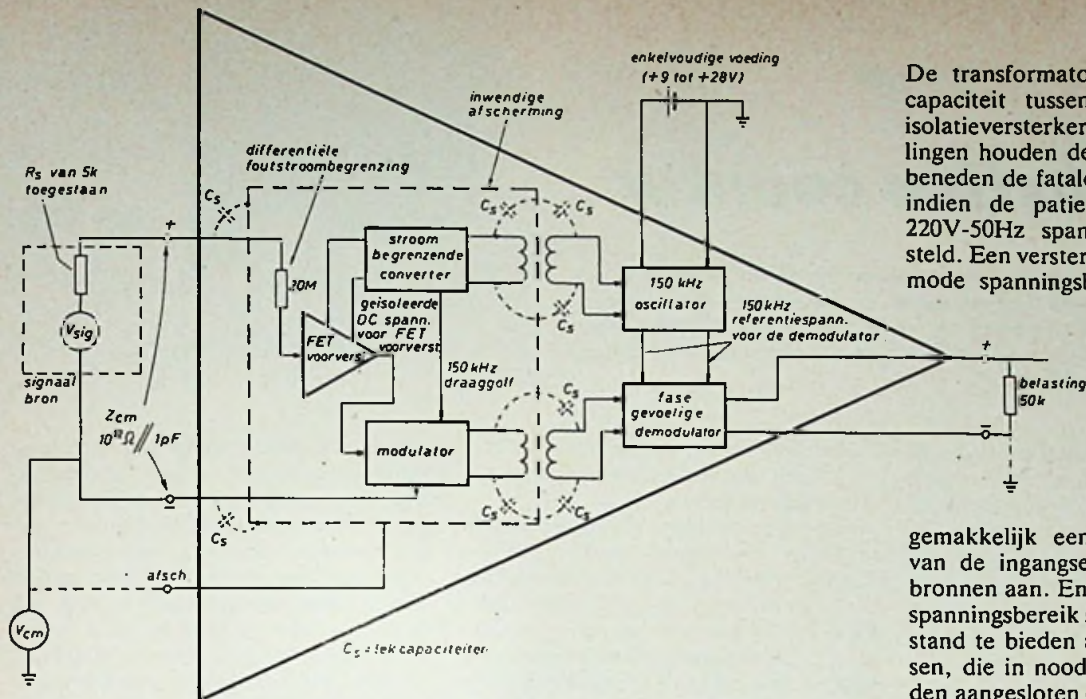
Fig. 5 Isolatie versterker van Analog Devices, model 272.
