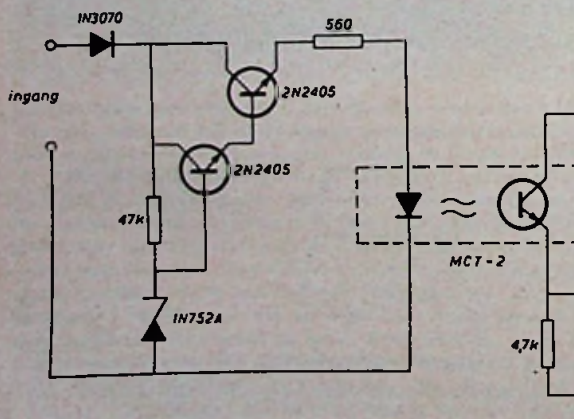
Fig. 5. Isolatie van twee digitale systemen. De Schmitt-trigger voorkomt ongewenste oscillaties.
