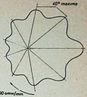
Fig. 25 Antenne patroon van het TACAN bakken.
