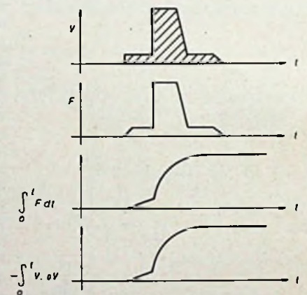
Fig. 1. Spanning naar frequentie omvormer als integrator.
