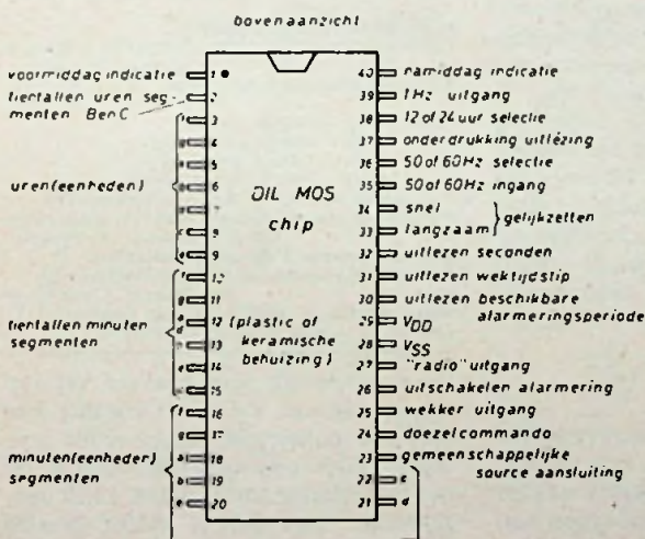
Fig. 7. Aansluitgegevens van de MOS klokchip.
