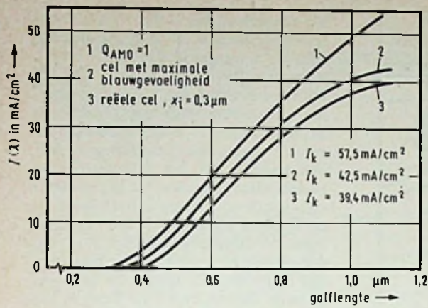
Fig. 6 Opgewekte stroom als functie van de golflengte voor een optimale cel, een cel met maximale blauwgevoeligheid en een reële cel.
