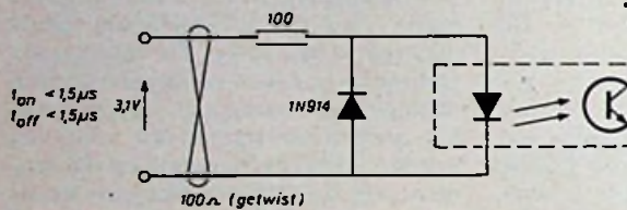
Fig. 2. Snelle lijnontvanger met de MCT 9.
