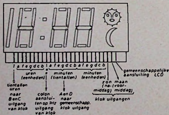
Fig. 4a. Transiiron LCD (T), in dit prototype toegepast.
