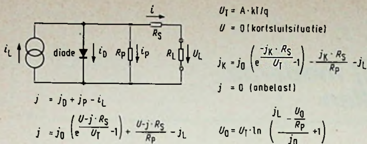
Fig. 3 Vervangingschema voor een silicium zonnecel.
